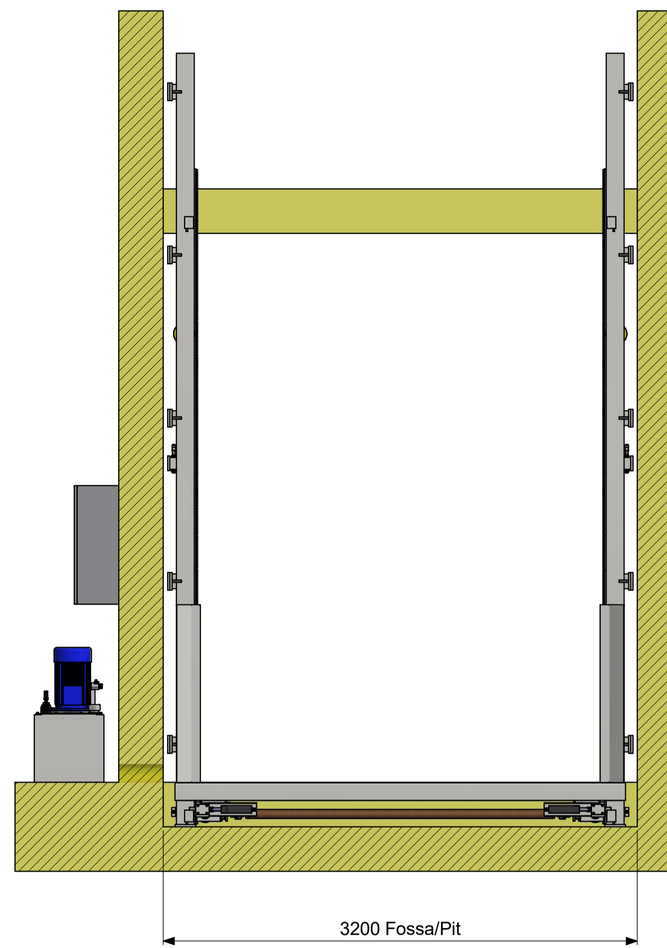
B-B ( 1 : 25 )
