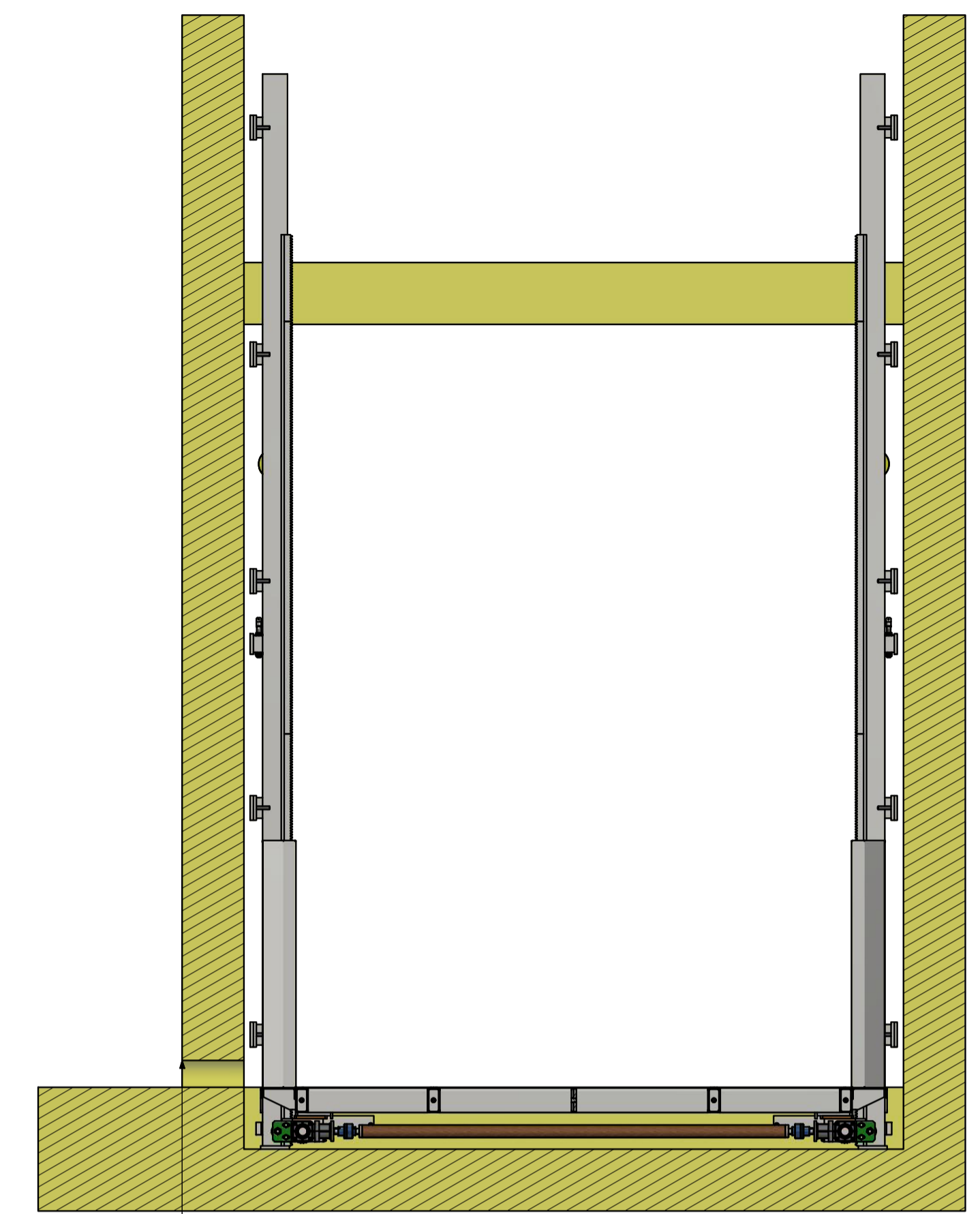
C-C ( 1 : 25 )
