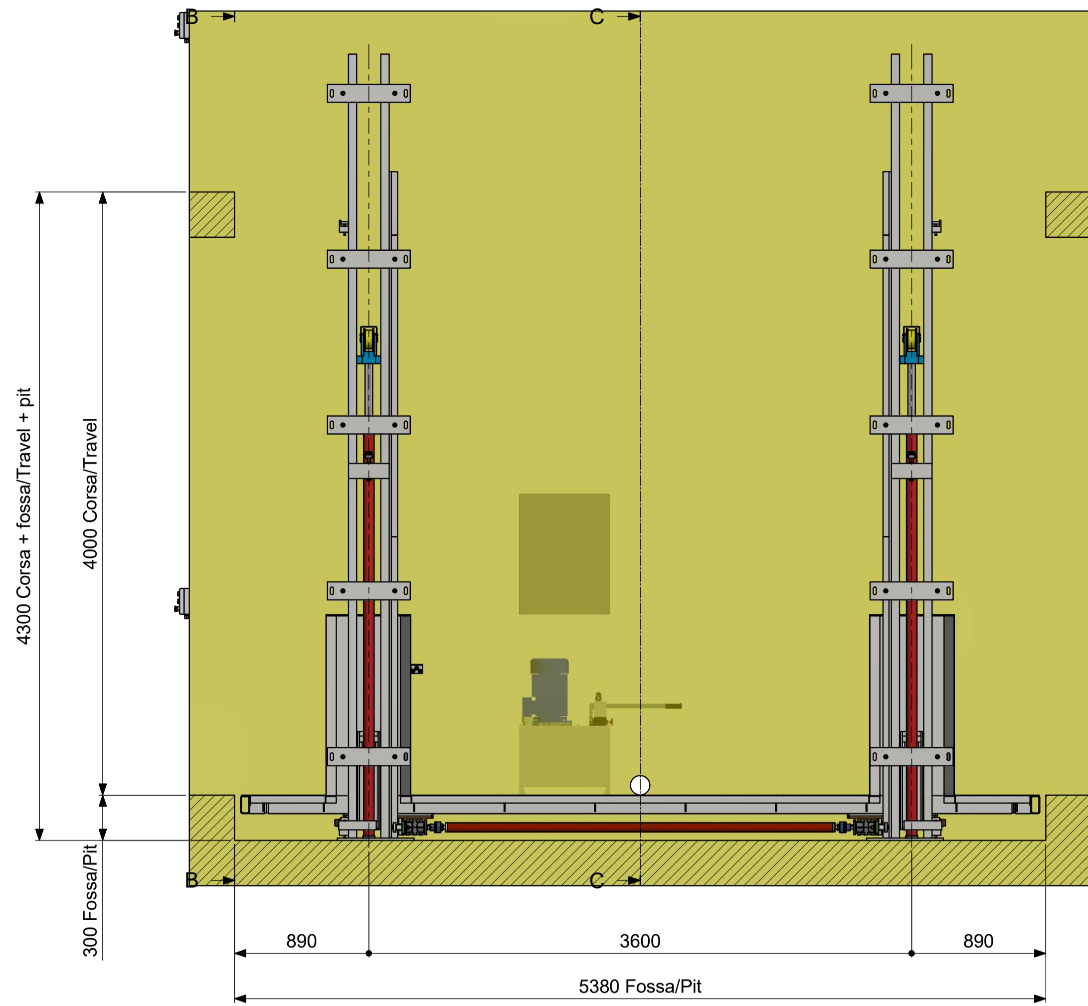
A-A ( 1 : 25 )
